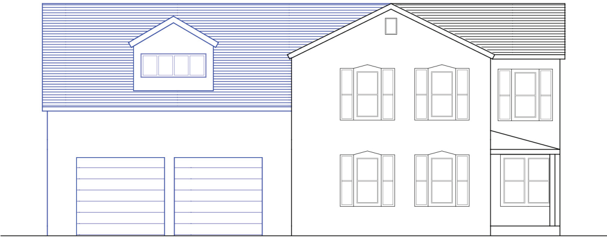
W. ELEVATION
