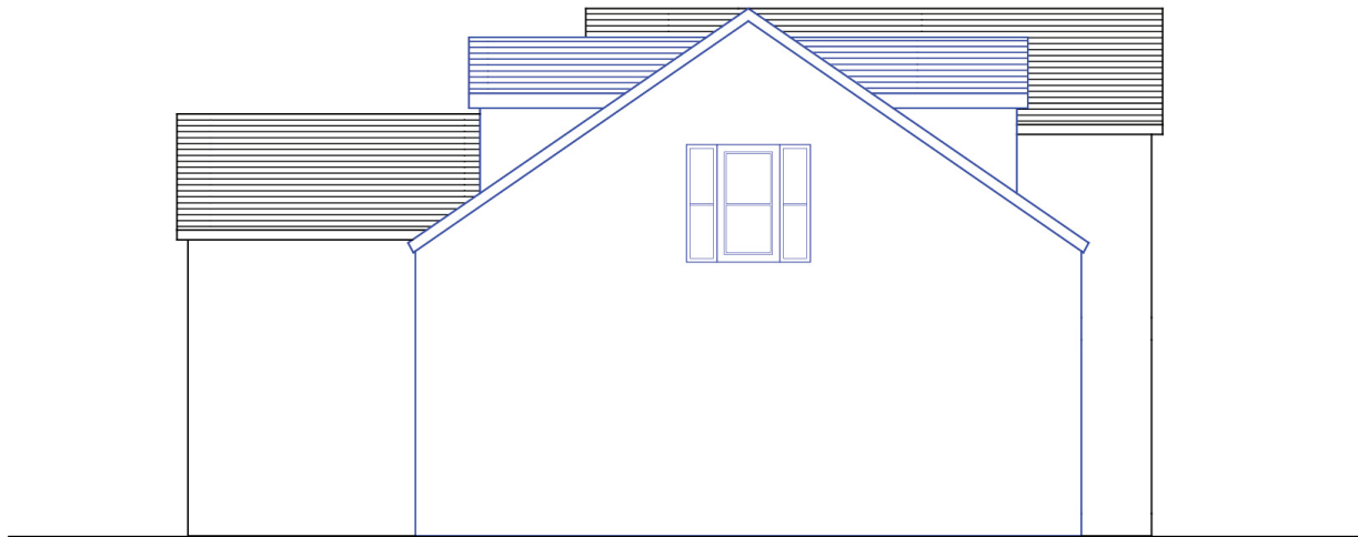
N. ELEVATION
